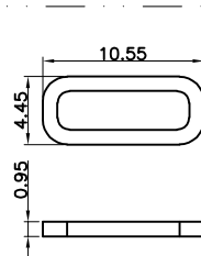
防水圈图示
